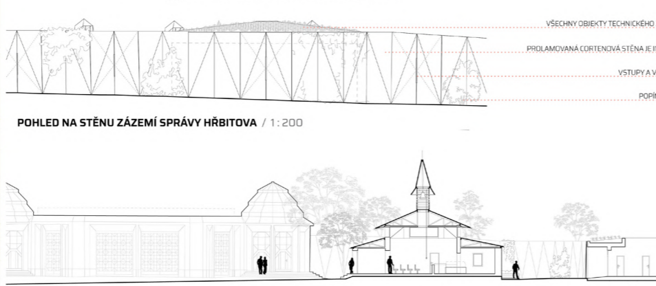
ŘEZ SMUTEČNÍ SÍNĚ A ZÁZEMÍ SPRÁVY HŘBITOVA / 1:200
