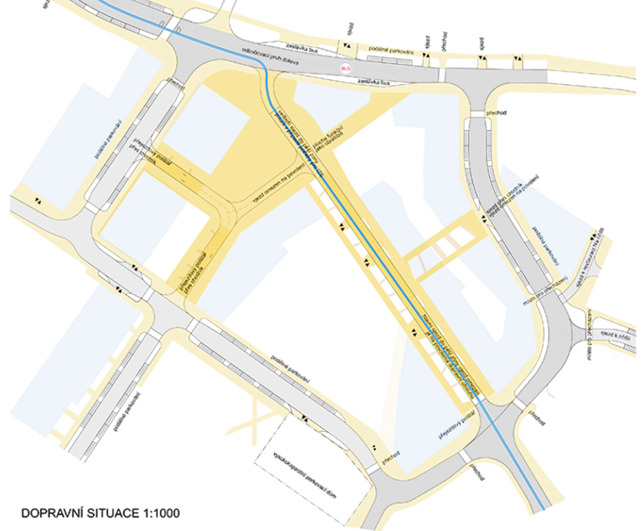
DOPRAVNÍ SITUACE 1:1000
