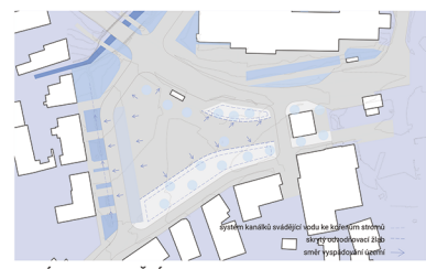
SCHEMA ODVODNĚNÍ
