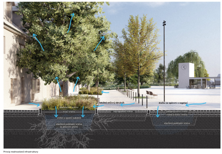
Principy podzemní infrastruktury
